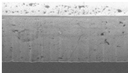
povrch stěny niklové planžety ( 150 um )
